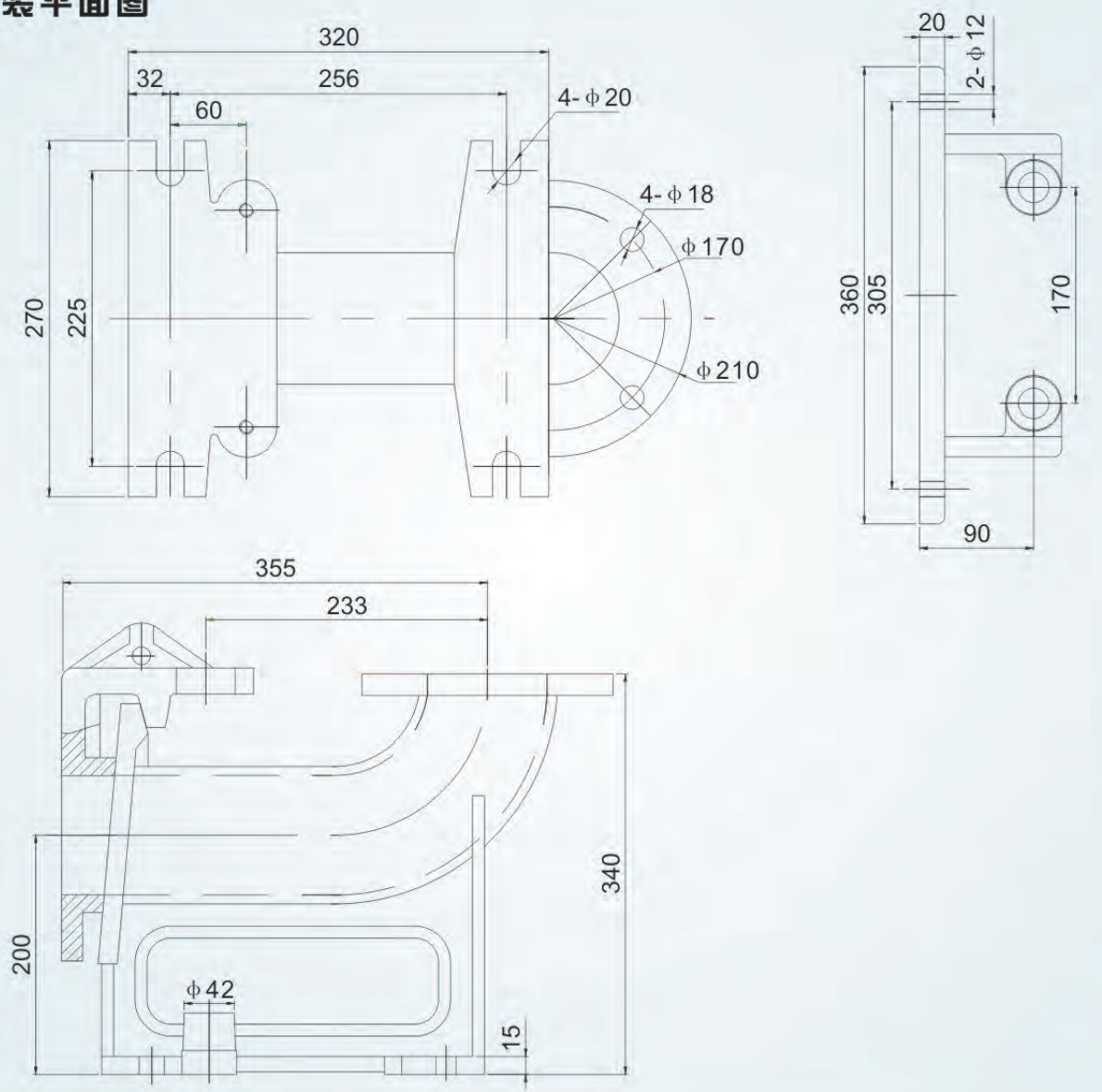
◆ 安装平面图
