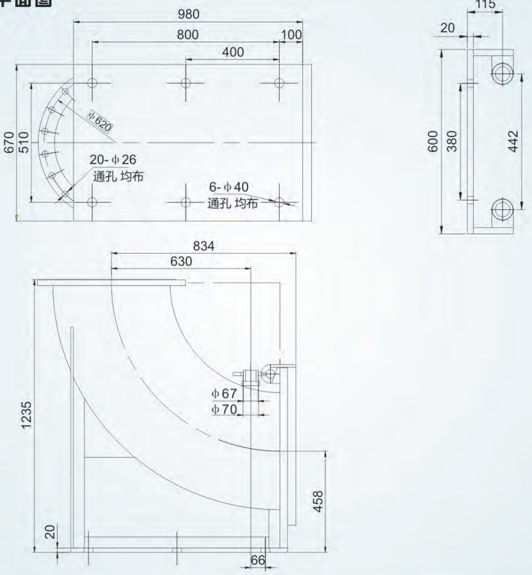
◆ 安装平面图
