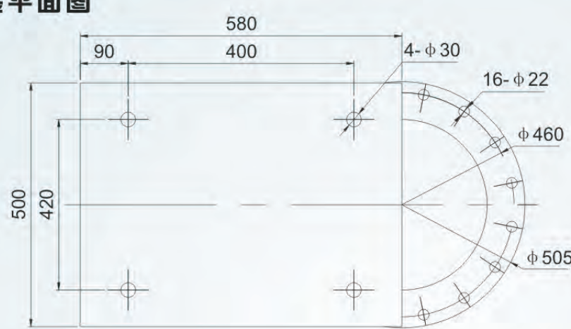
◆ 安装平面图
