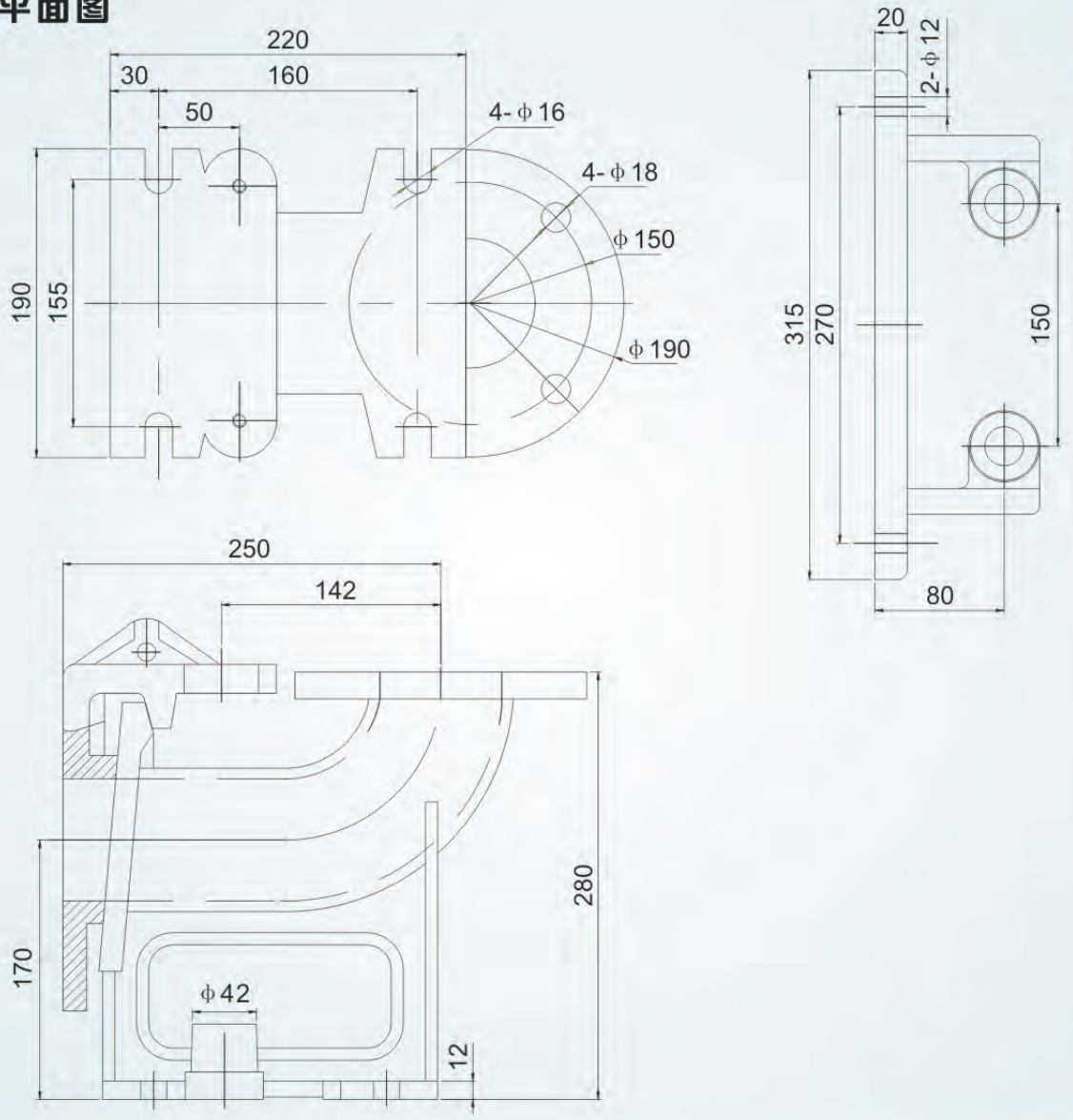
◆ 安装平面图
