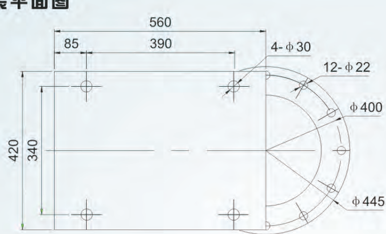
◆ 安装平面图
