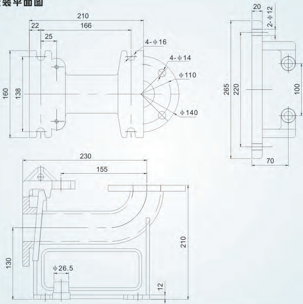
◆ 安装平面图
