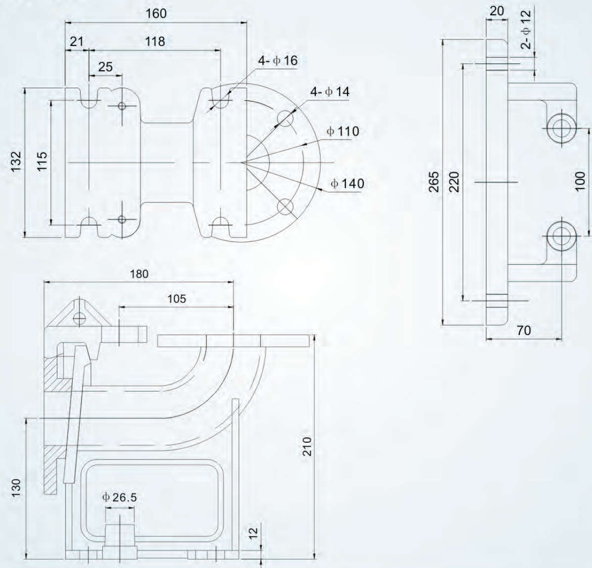
◆ 安装平面图
