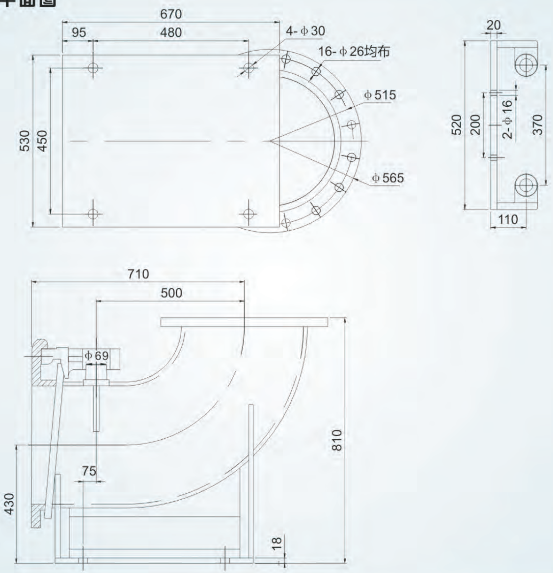
◆ 安装平面图
