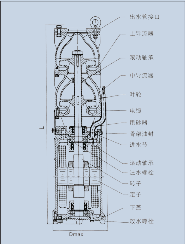
外形型尺寸图
