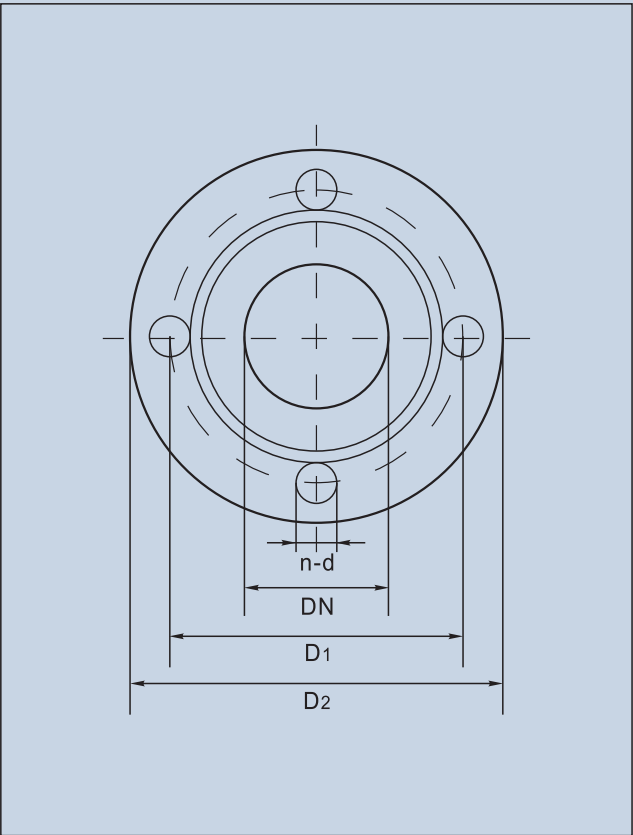
出口法兰尺寸图
