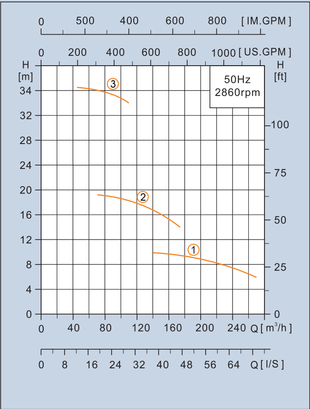
性能曲线
