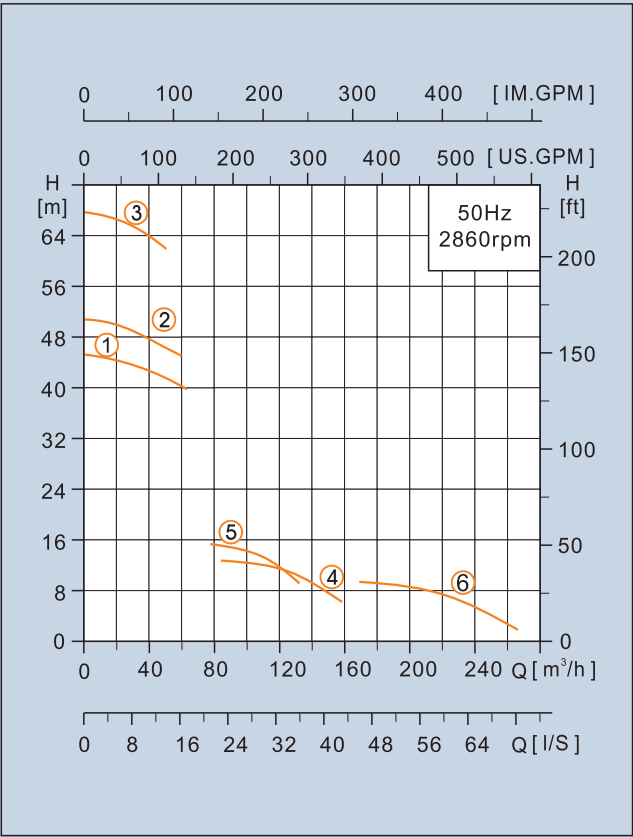
性能曲线
