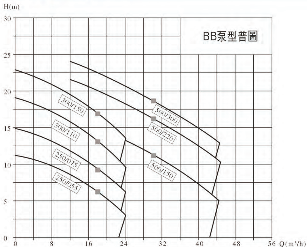
BB泵型普圖 BB Pump Curves
